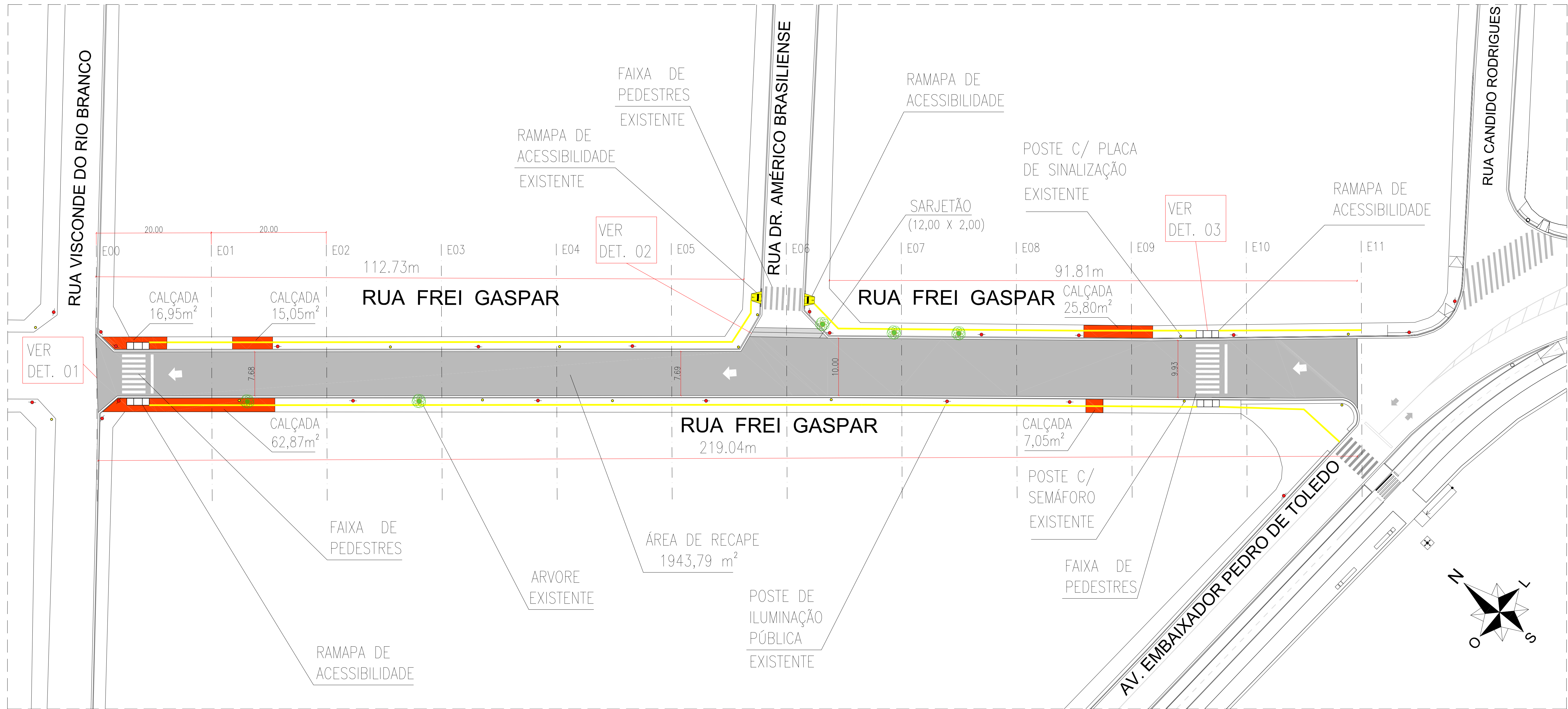
SITUAÇÃO -PROJETADA-RECAPE RUA FREI GASPAR SEM ESCALA
