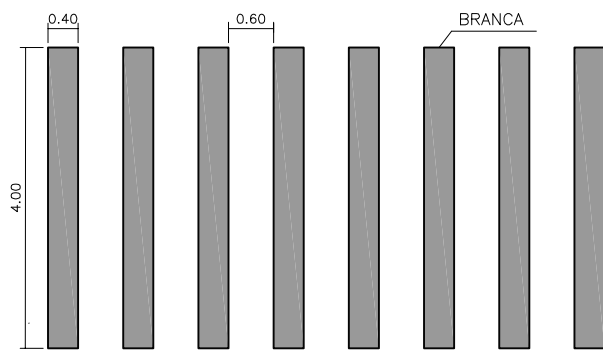
SINALIZAÇÃO HORIZONTAL DETALHE - FAIXA DE PEDESTRE ESCALA 1:50
