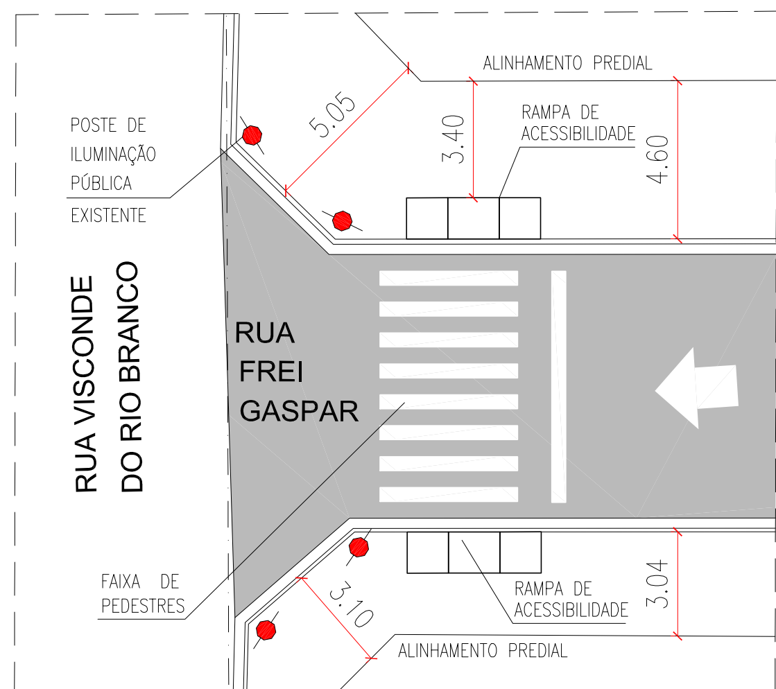
DETALHE 01 RUA FREI GASPAR SEM ESCALA
