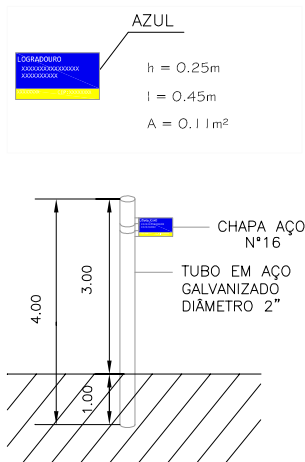
DETALHE - PLACAS DE LOGRADOURO S/ ESCALA
