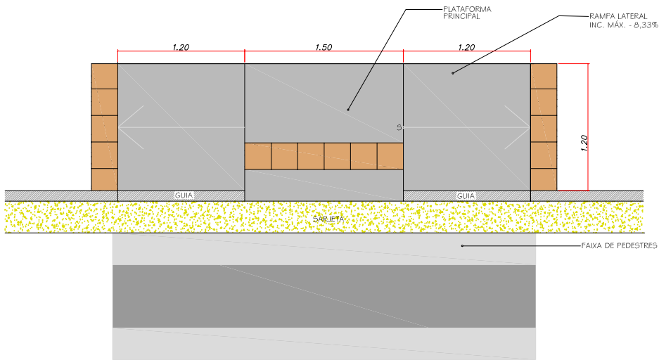
DETALHE - RAMPA ACESSIBILIDADE ESCALA 1:50
