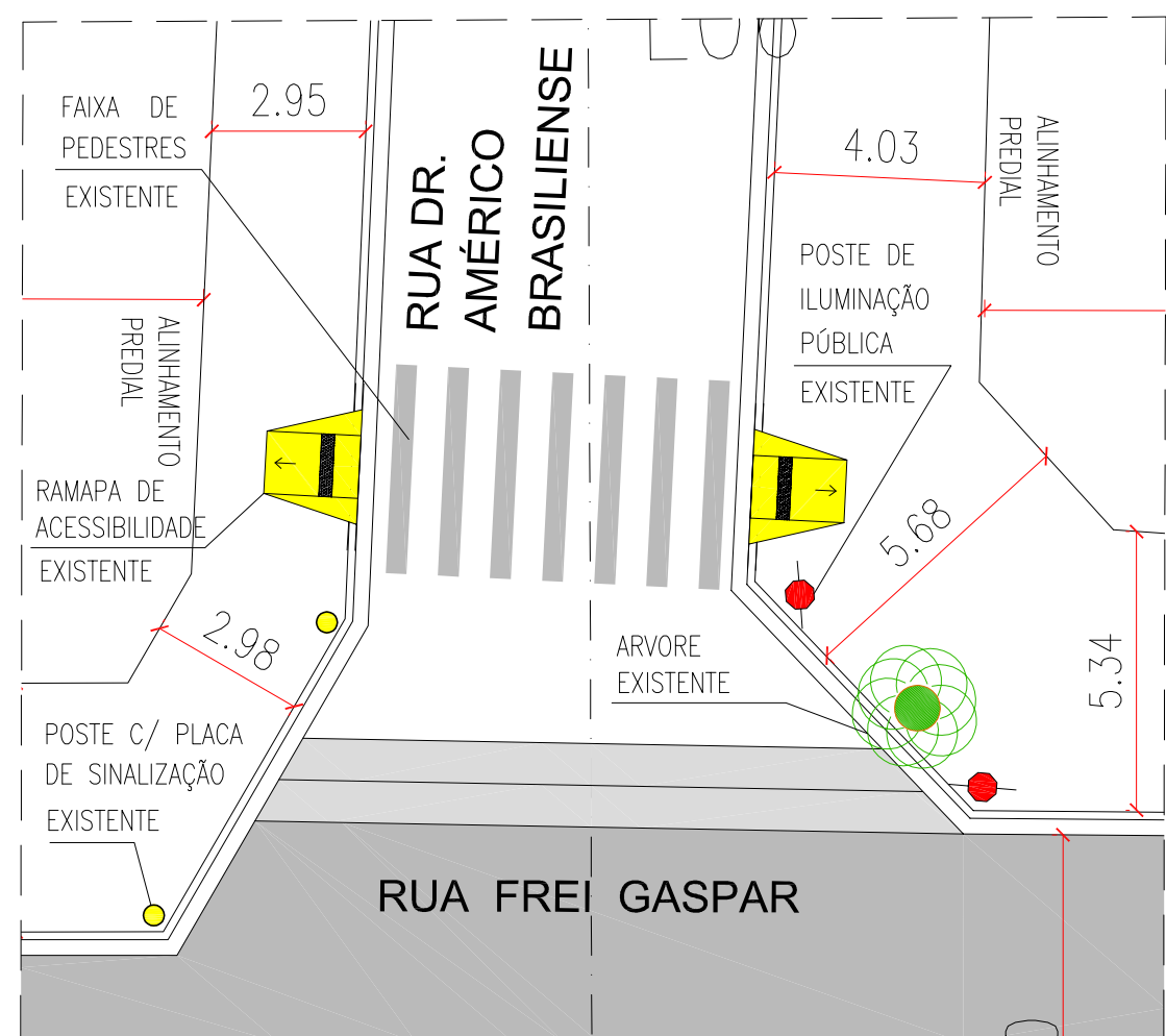
DETALHE 02 RUA FREI GASPAR SEM ESCALA
