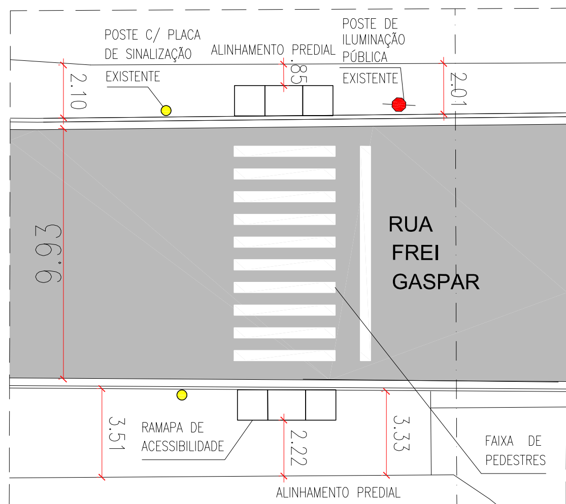
DETALHE 03 RUA FREI GASPAR SEM ESCALA
