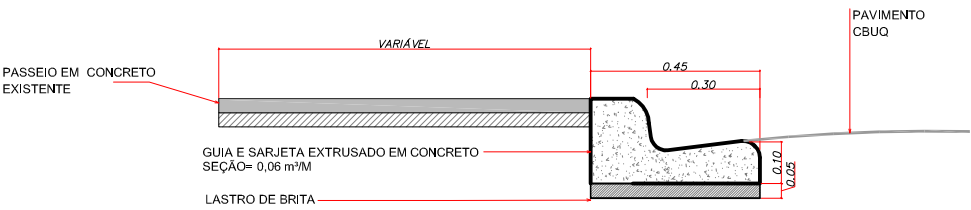
DETALHE - PERFIL EXTRUSADO ESCALA 1:20
