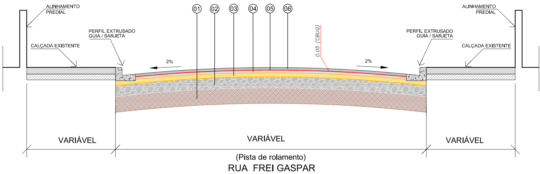
SEÇÃO TÍPICA DO PAVIMENTO ESCALA 1:50
