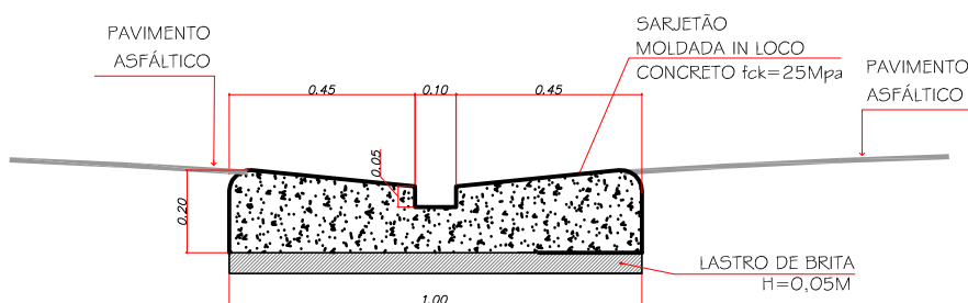
DETALHE - SARJETÃO ESCALA 1:20
